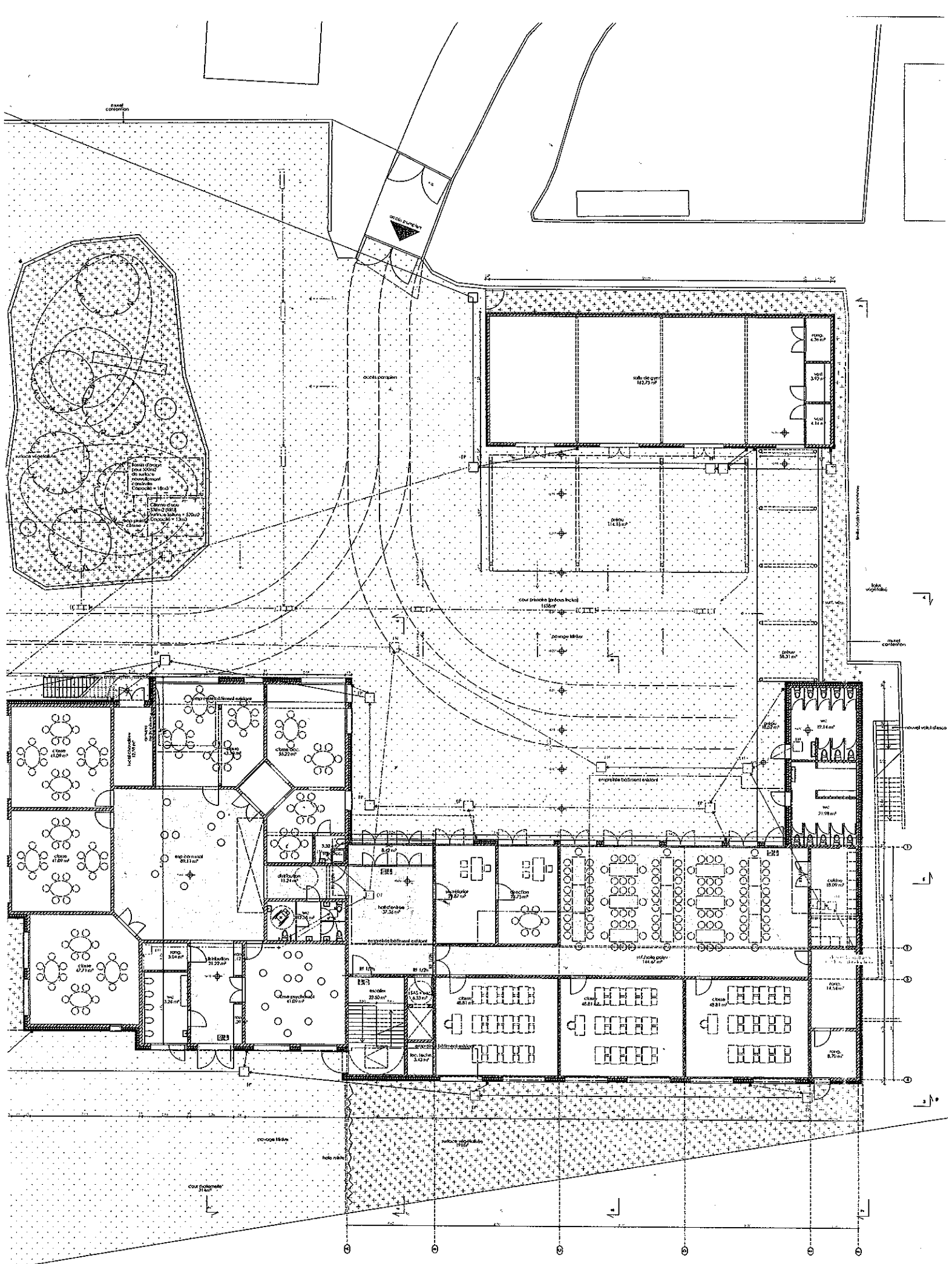
PLAN RDC - SITUATION PROJETEE Echelle 1/100 ème
